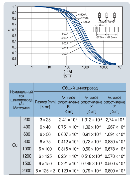
Рис. 10. Понижающий коэффициент для общей шины (медной)
