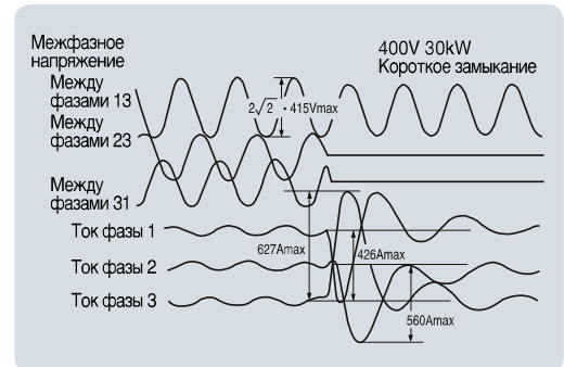
Рис.2. Короткое замыкание электродвигателя
